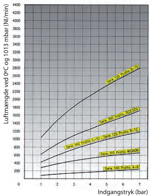
Flow karakteristisk med 1 bar tryktab
