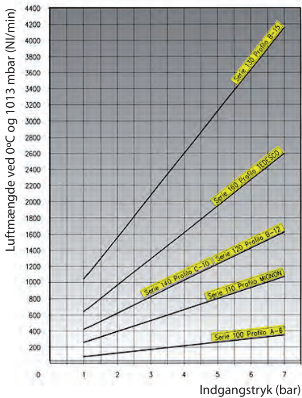
Flow karakteristisk med udstødning til atmosfære
